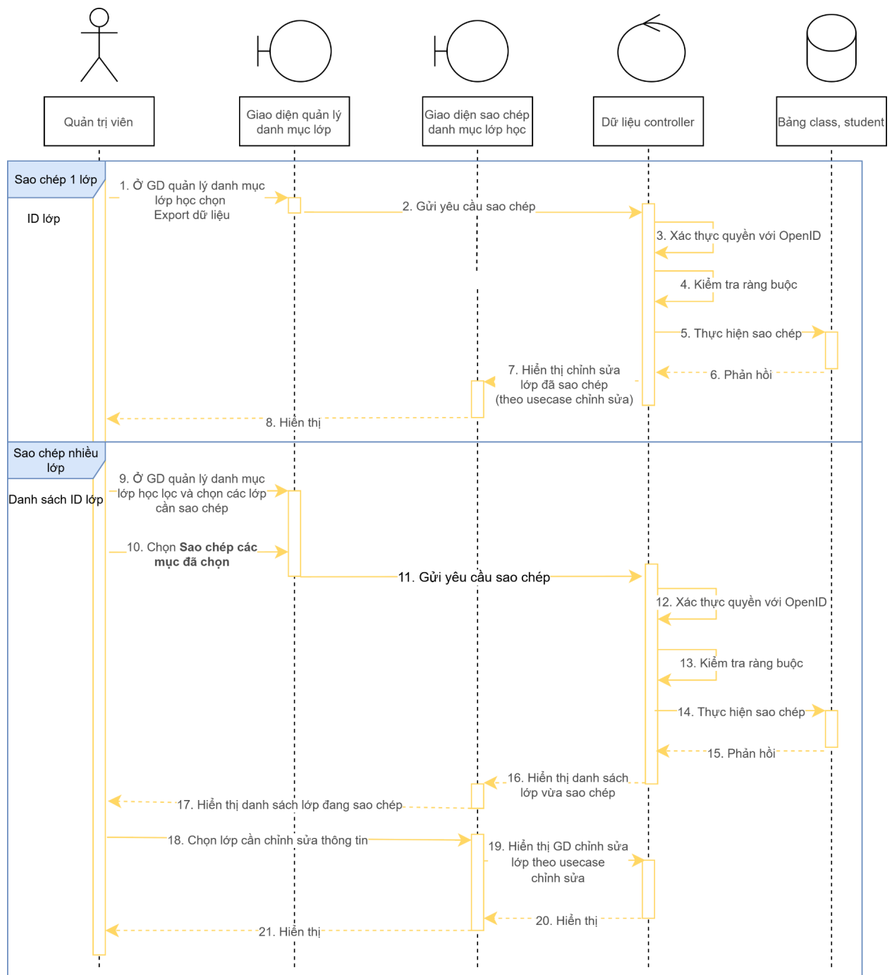
Figure 23. Sơ đồ trình tự usecase sao chép lớp học
